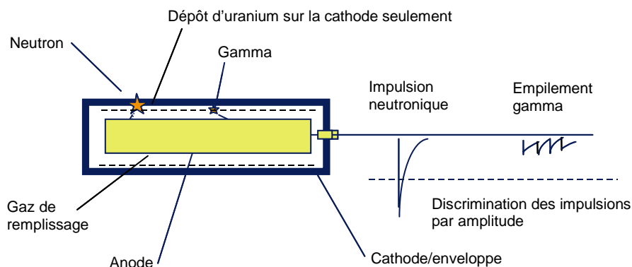
Figure 4 – Schéma d'un compteur à fission
