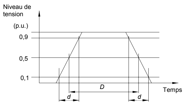
Figure 2b - Onde d'essai
