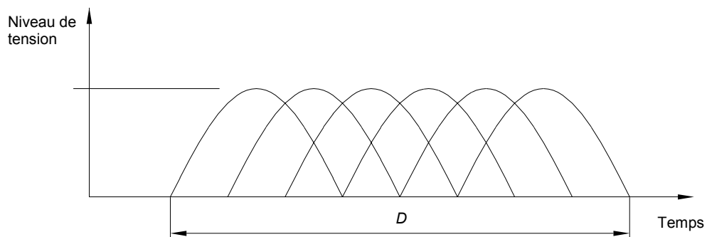
Figure 3b - Forme d'onde d'essai
