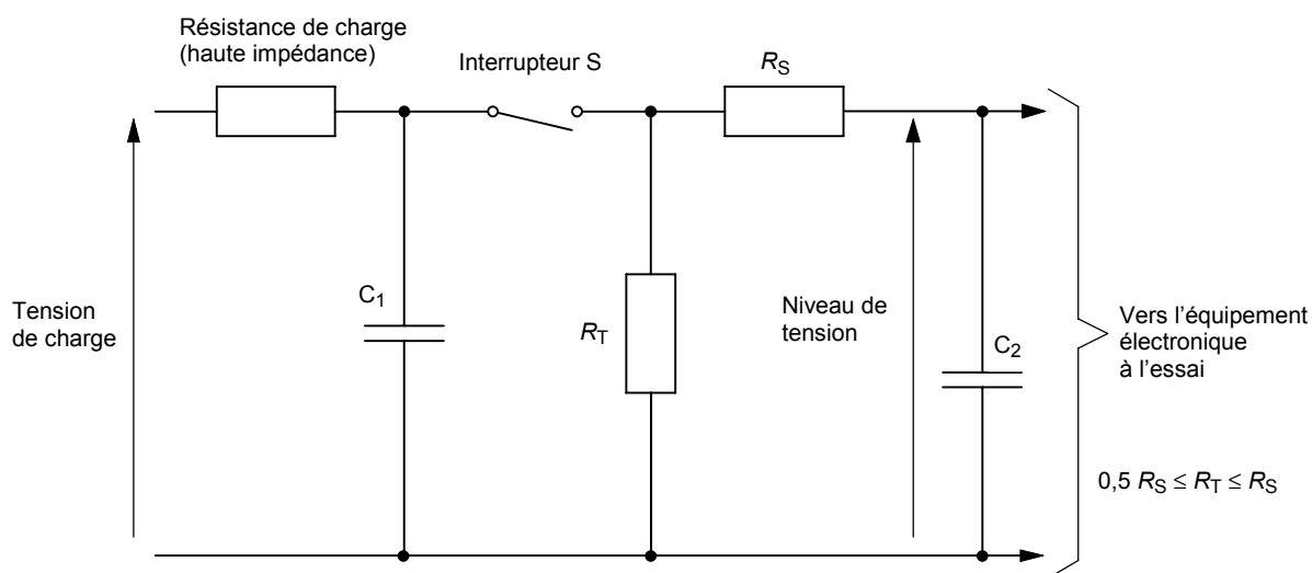
Figure 4a - Circuit d'essai
