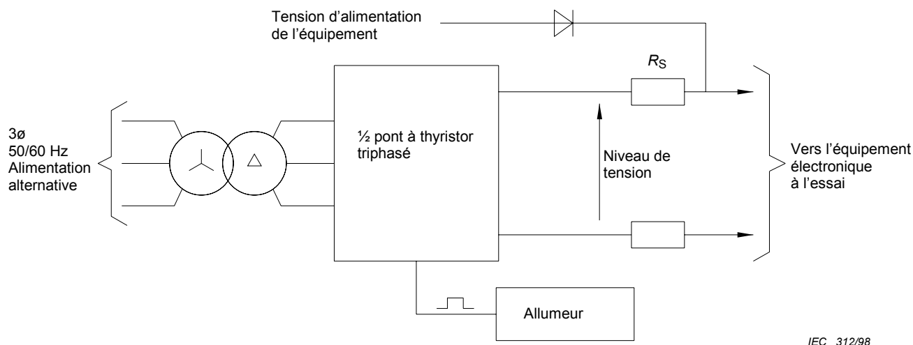
Figure 3a - Circuit d'essai type
