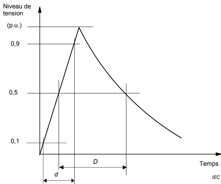
Figure 4b - Forme d'onde d'essai
