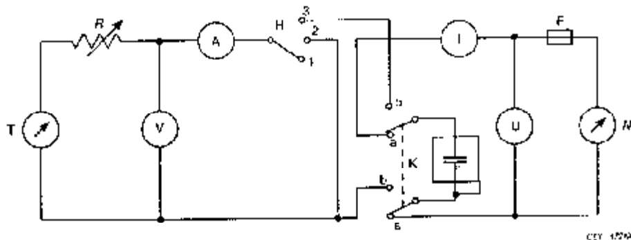
Figure 1 – Circuit pour réaliser l'essai de destruction
