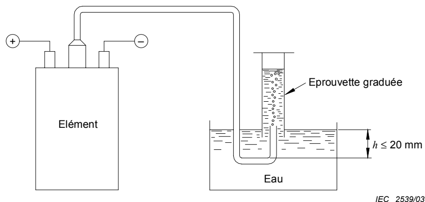
Figure 1 – Méthode de collecte de gaz
